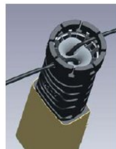
Konstrukce základny umožňuje instalovat PE trubky do 8 různých poloh
